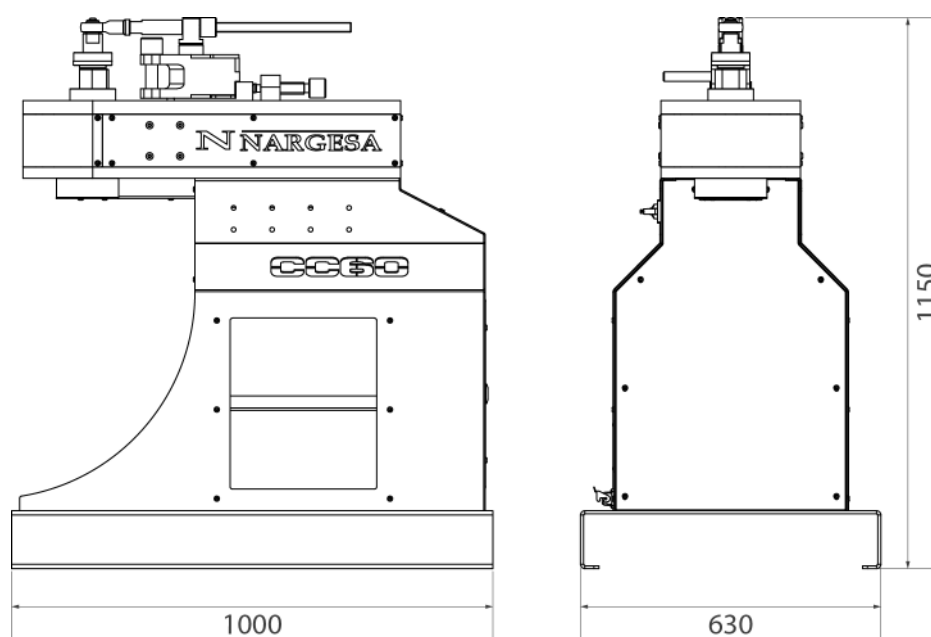
Figura 1. Dimensiones exteriores de la Curvadora CC60
