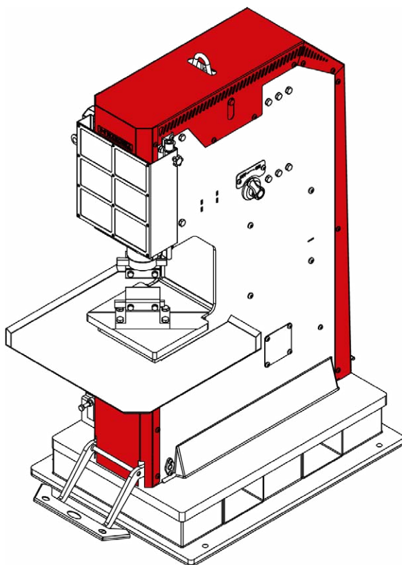
Figura 3. Resguardos de protección del Martillo Pílon
