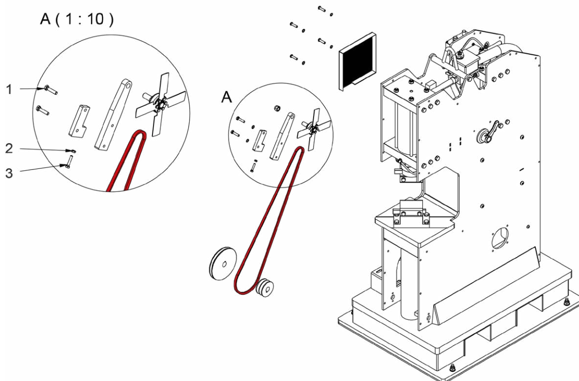
Figura 6. Correa del ventilador
