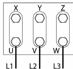
Figura 10. Figura triángulo para tensión 220V
