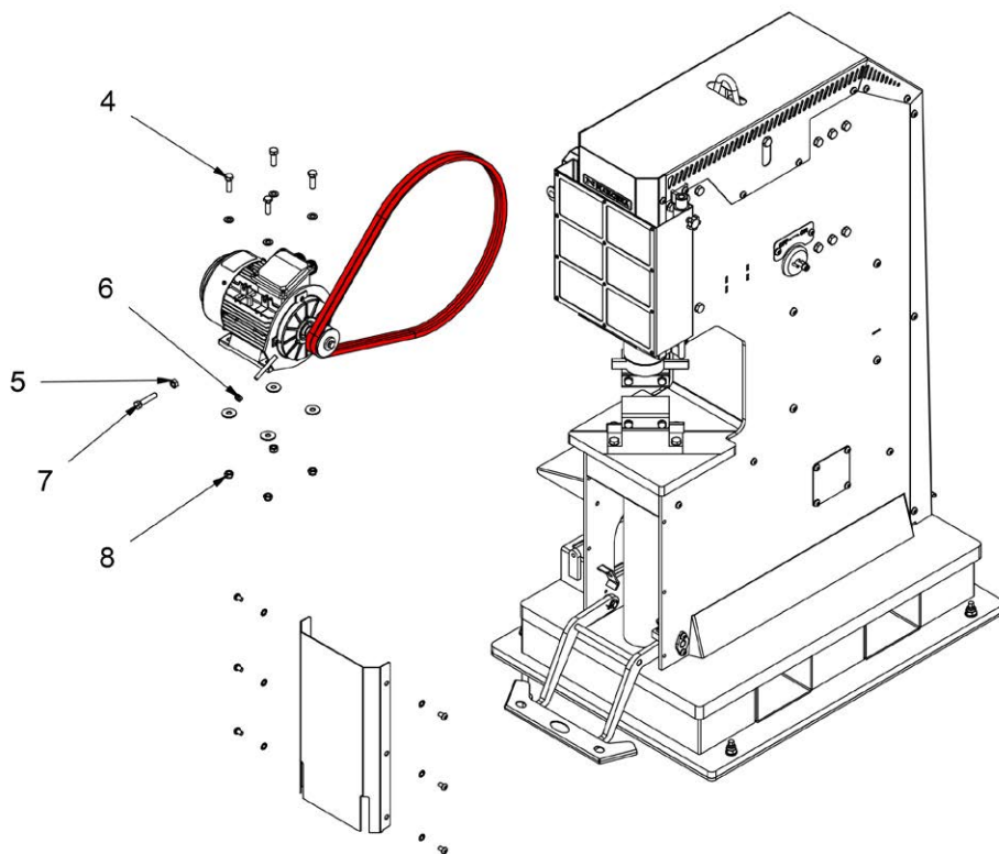
Figura 7. Correas del accionamiento principal
