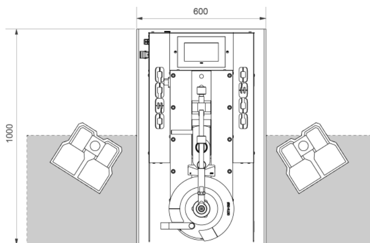
Figura 6. Zona de trabajo del operario
