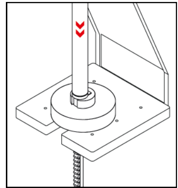
6. Bajar pistón
