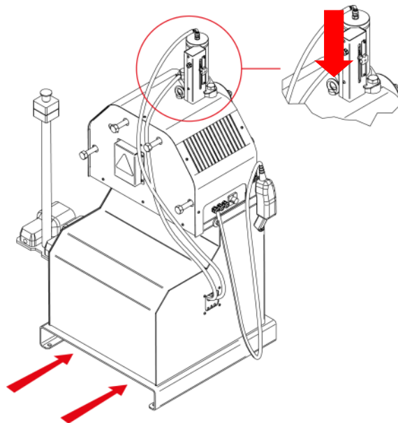
Figura 4. Transporte de la máquina
