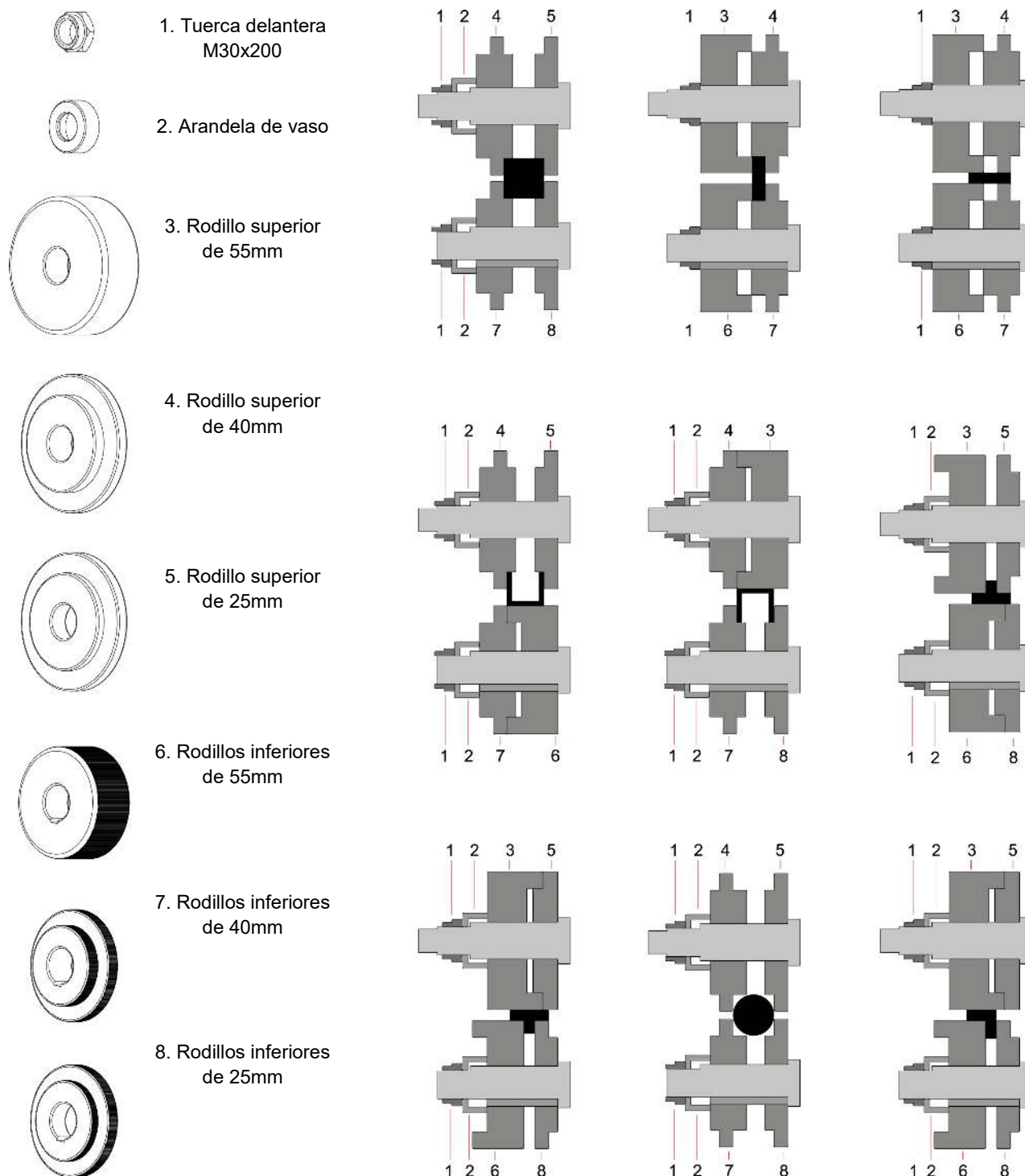
Figura 15. Nomenclatura de los rodillos y ensamble
