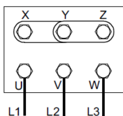
Figure en étoile (prédéterminée) Pour tension 400V
