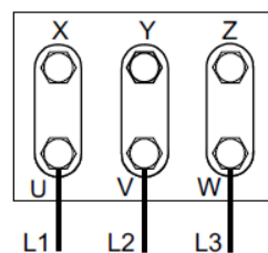
Figure 11. Figure triangle pour tension 230V
