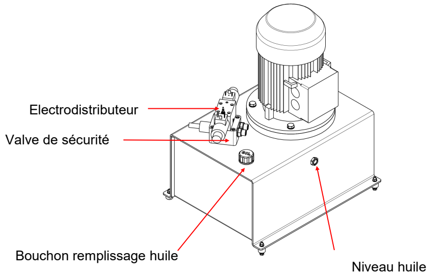
Figure 5. Identification des composants du réservoir hydraulique
