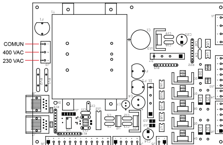
Figure 12. Emplacement du borne 6 sur la plaque électrique
