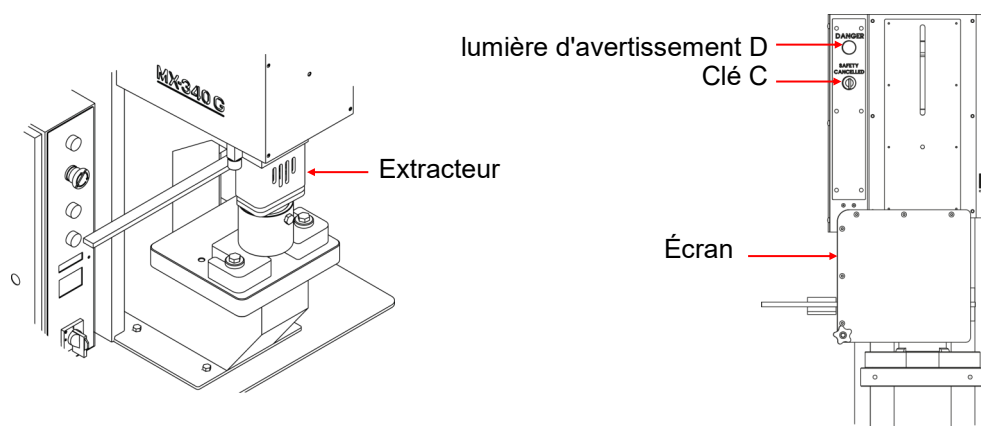
Figure 3. Protections de la poinçonneuse
