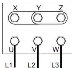
Figure 10. Figure étoile pour tension 400V (prédéterminé)
