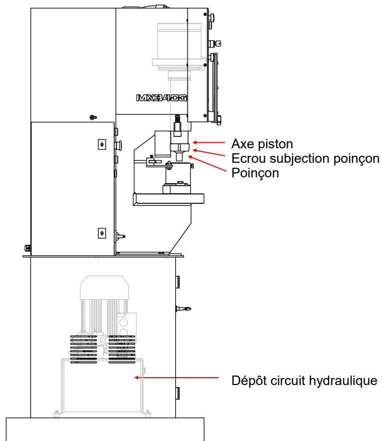
Figure 2. Nomenclature des composants de la machine
