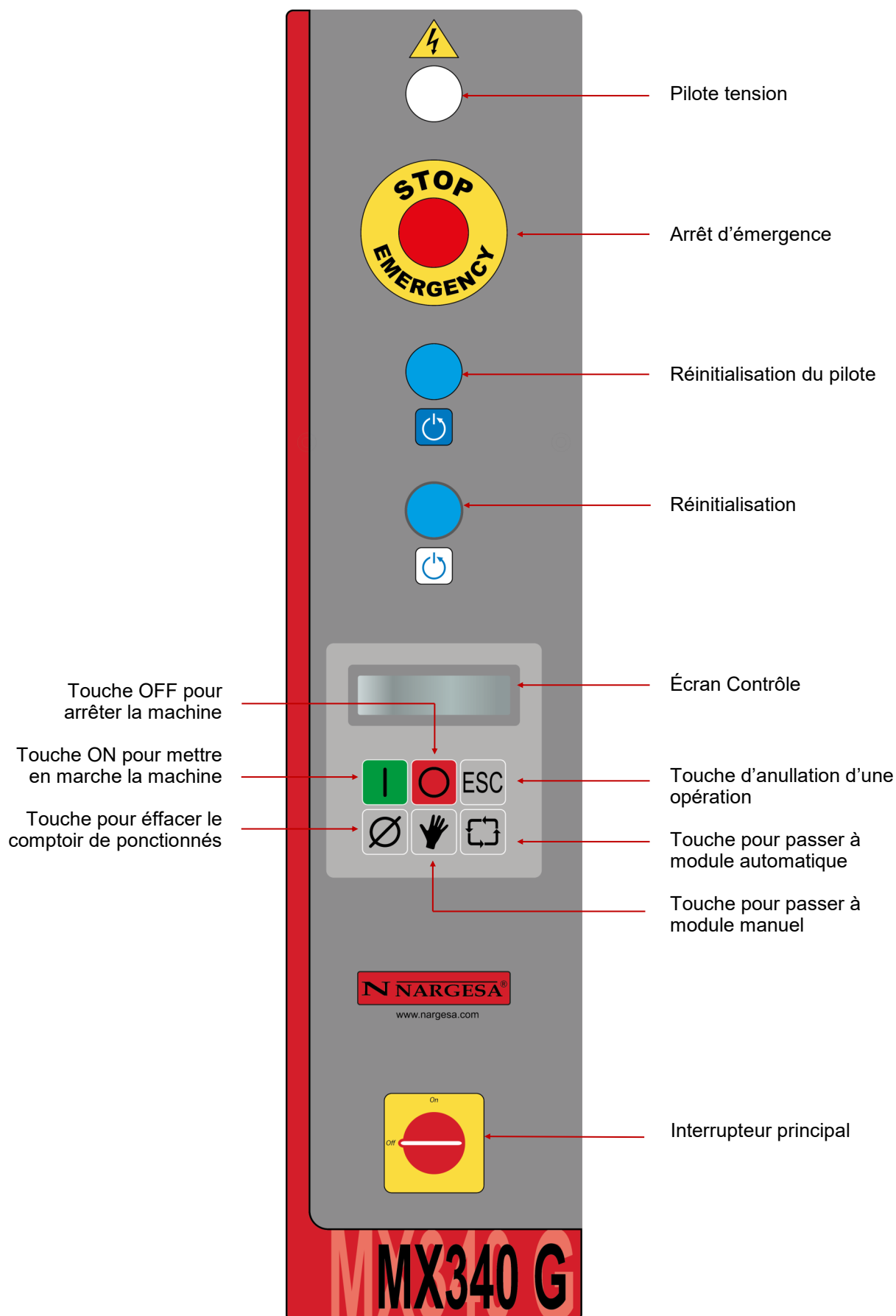
Figure 13. Panneau de commande
