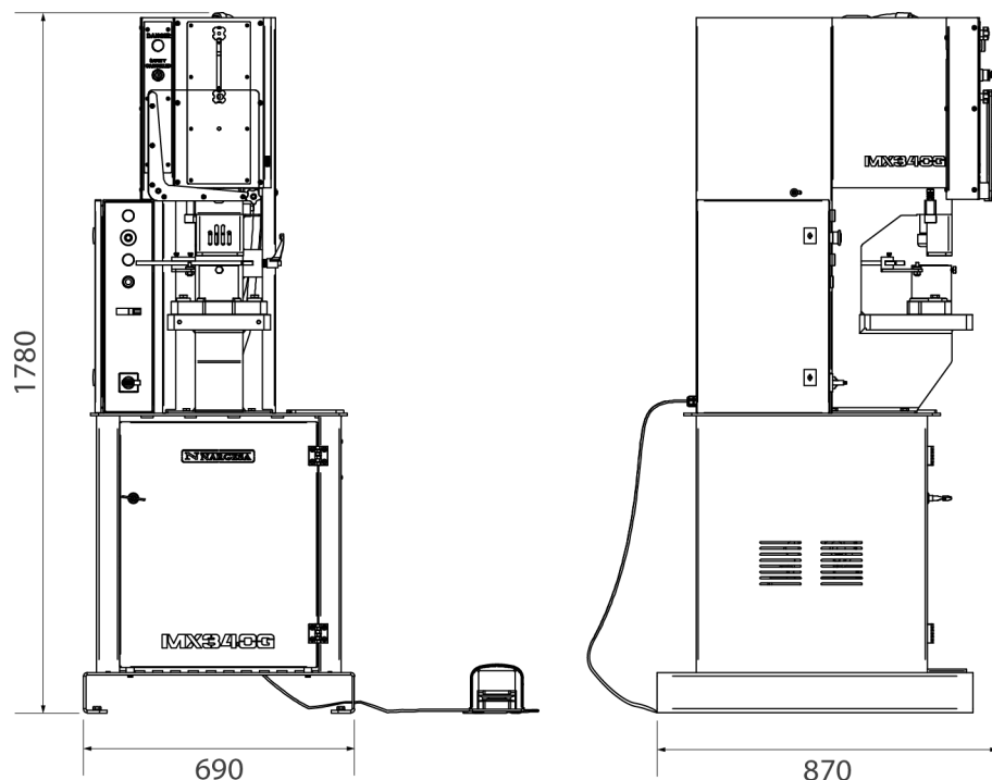
Figure 1. Dimensions extérieures de la poinçonneuse MX340G
