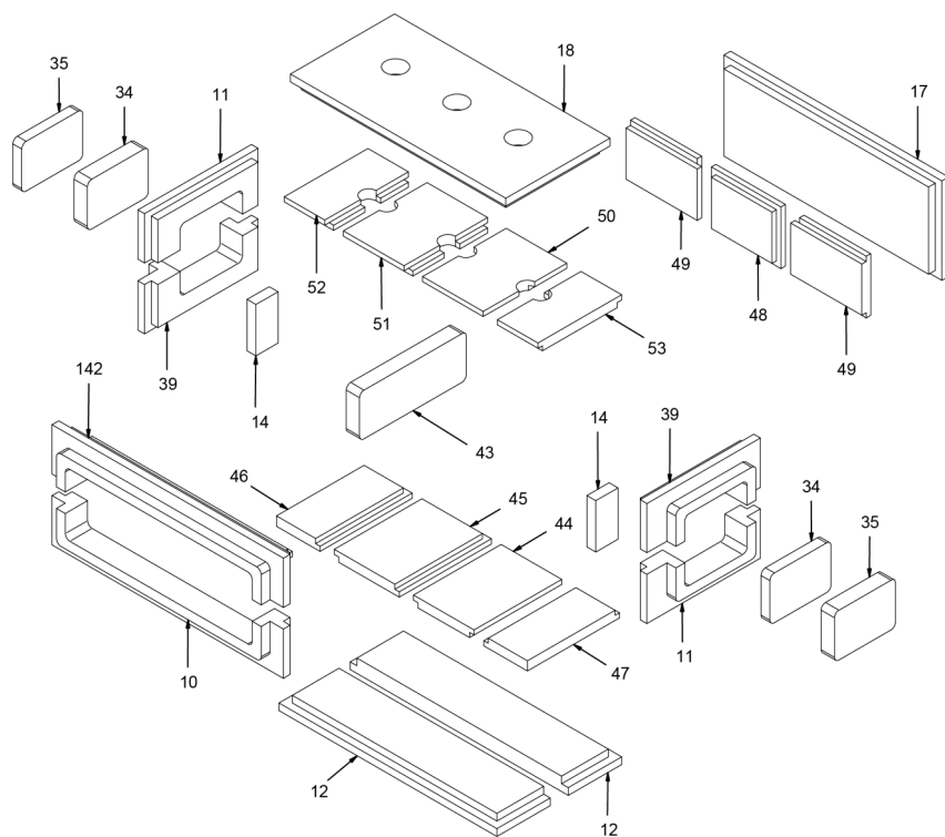
Image 7. Kit de matériel isolant
